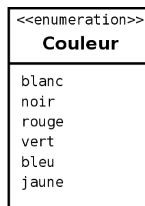
FIG. 4.9 – Définition d'une énumération en utilisant un classeur.
