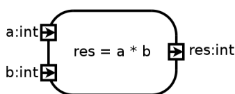
FIG. 6.7 – Représentation des pins d'entrée et de sortie sur une activité.
